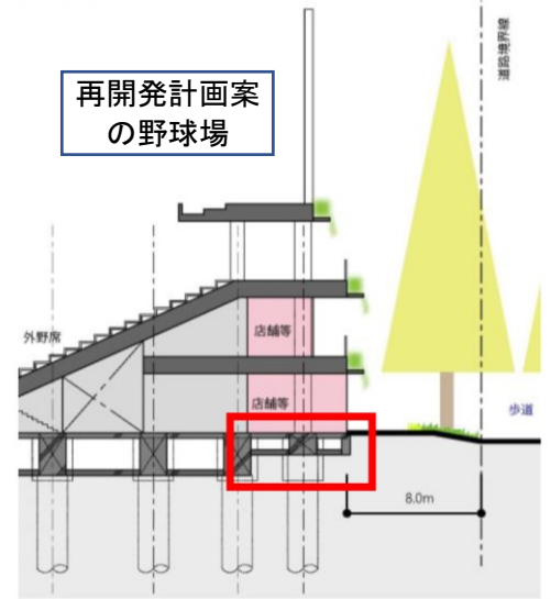
いちよう並木側の基礎梁については、扁平化する等 考慮し、掘削範囲の低減に配慮して継続検討
